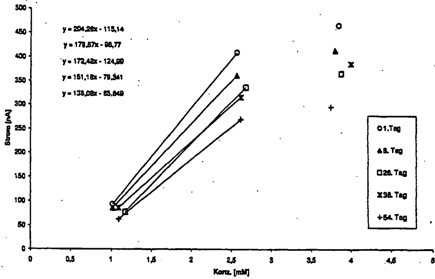
Abbildung 7: Sensitivität von ADPA-modifizierten Glukosebiosensoren ohne Schutzschicht in Abhängigkeit des Sensoralters
